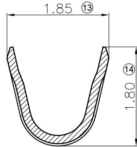
SECTION A-A SCALE 15:1
